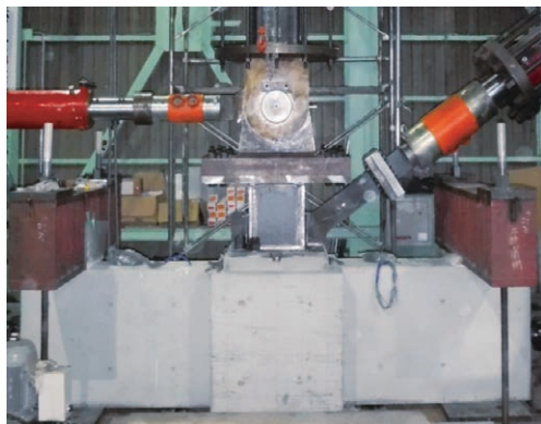
実験風景
