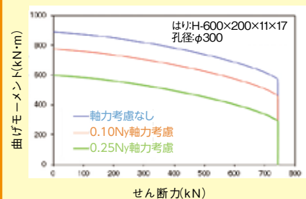
耐力図
