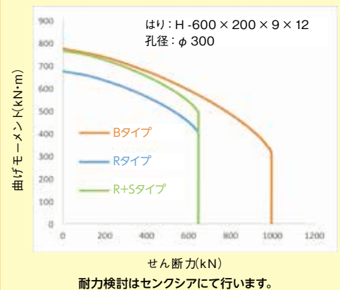
R,B,R+S タイプの耐力図例
