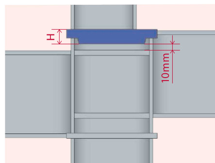
はり段差がある場合、内ダイアフラムとスマートダイアの距離を10mm以上確保
