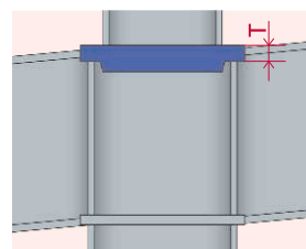
はりフランジがスマートダイア側面に取り付くことを確認（T寸法の範囲内）
