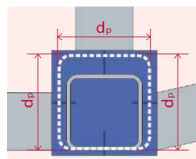
はりフランジが下階柱の外側よりも内側に取り付くことを確認（ d_p 寸法の範囲内）
