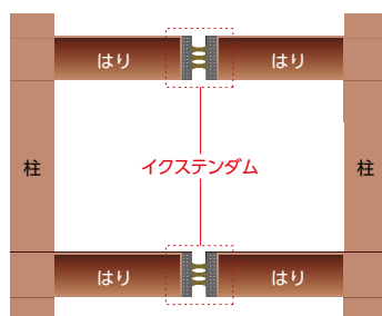
■はり設置型
