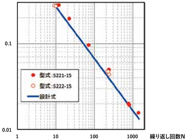
図3 疲労特性
