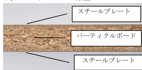
ウッドコアスチールフロア断面
