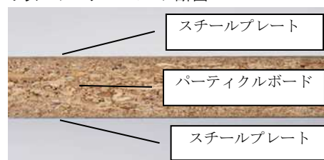
ウッドコアスチールフロア断面
